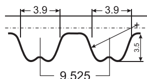
Профиль ремней ГРМ 2108-1006040 и 2112-1006040
