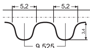
Профиль ремней ГРМ 21126-1006040
